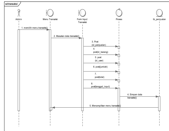
Gambar 5. Sequence Diagram Transaksi Penjualan
