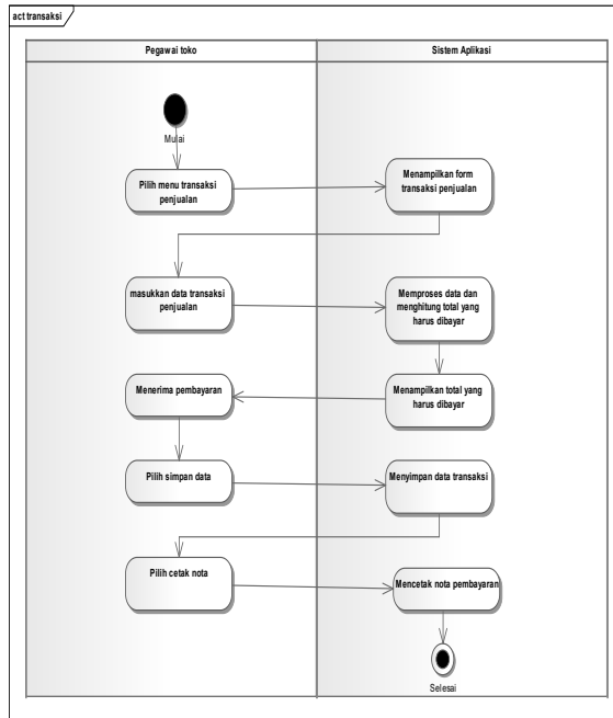
Gambar 3. Activity Diagram Transaksi Penjualan
